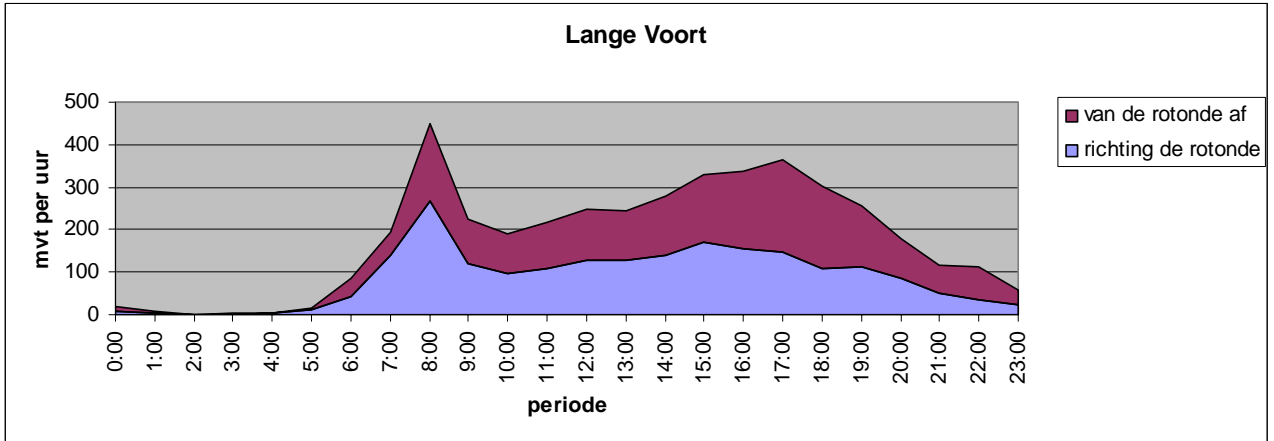
Figuur 2.1: verdeling aantal motorvoertuigen over een werkdag (telcijfers van 31/01/05 – 04/02/05)
